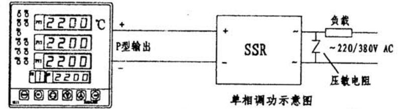
单相调功示意图
