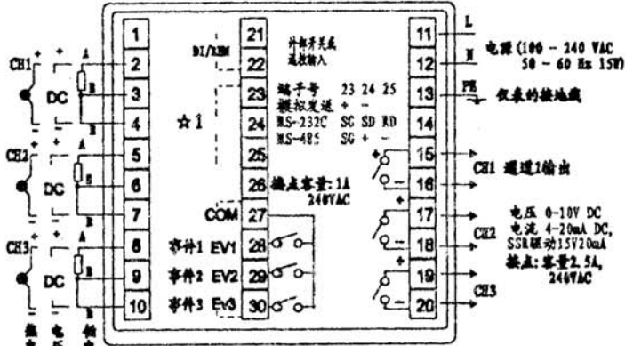
MR13 端子接线图
