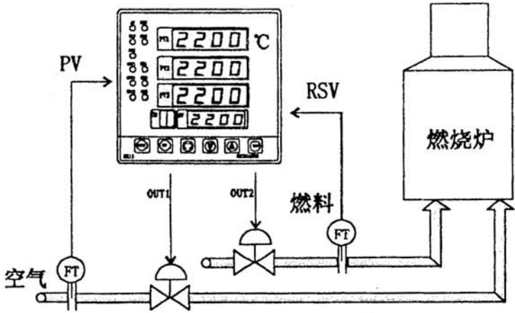
MR13的比值调节
