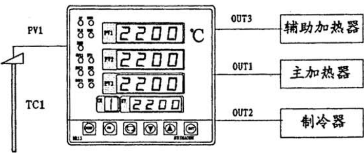
MR13的主辅调节或正反调节输出
