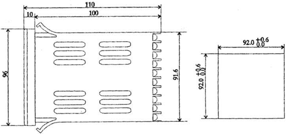
MR13外形及开口尺寸
