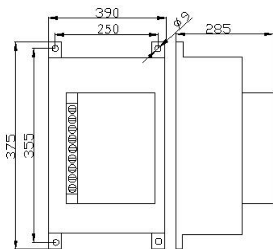
图 I (B400 散热器)
