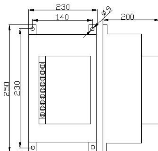
图 I (B227 散热器)
