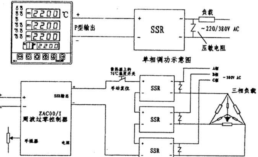
三相调功示意图(中心不接地可采用两控三相方案)
