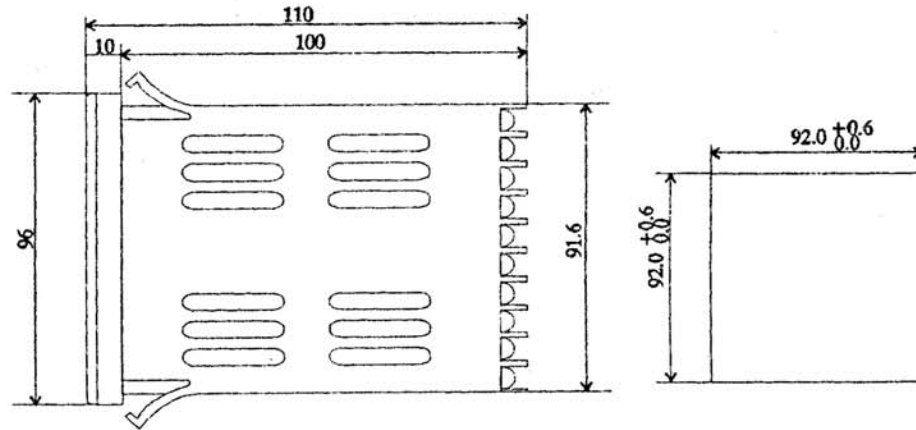
MR13外型及开口尺寸
